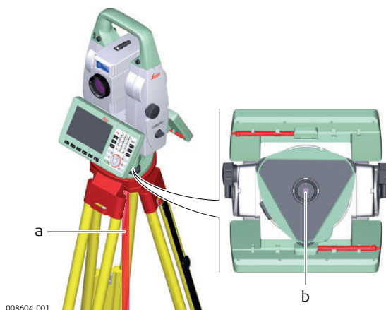
008604.001 а) Лазерный луч б) Выход лазерного луча
